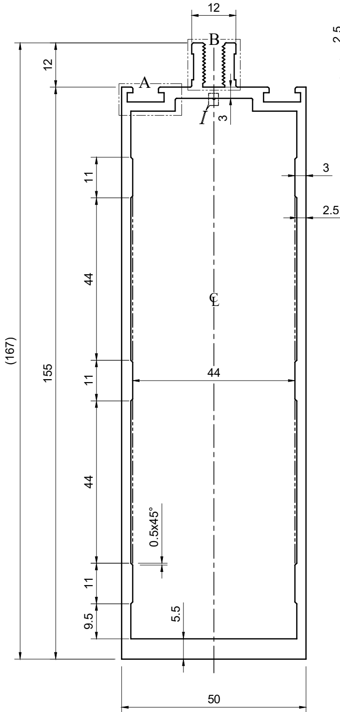
SCALE 1:1
